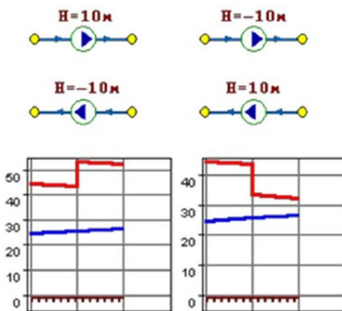
Рисунок 3.2.15. Пьезометрические графики
