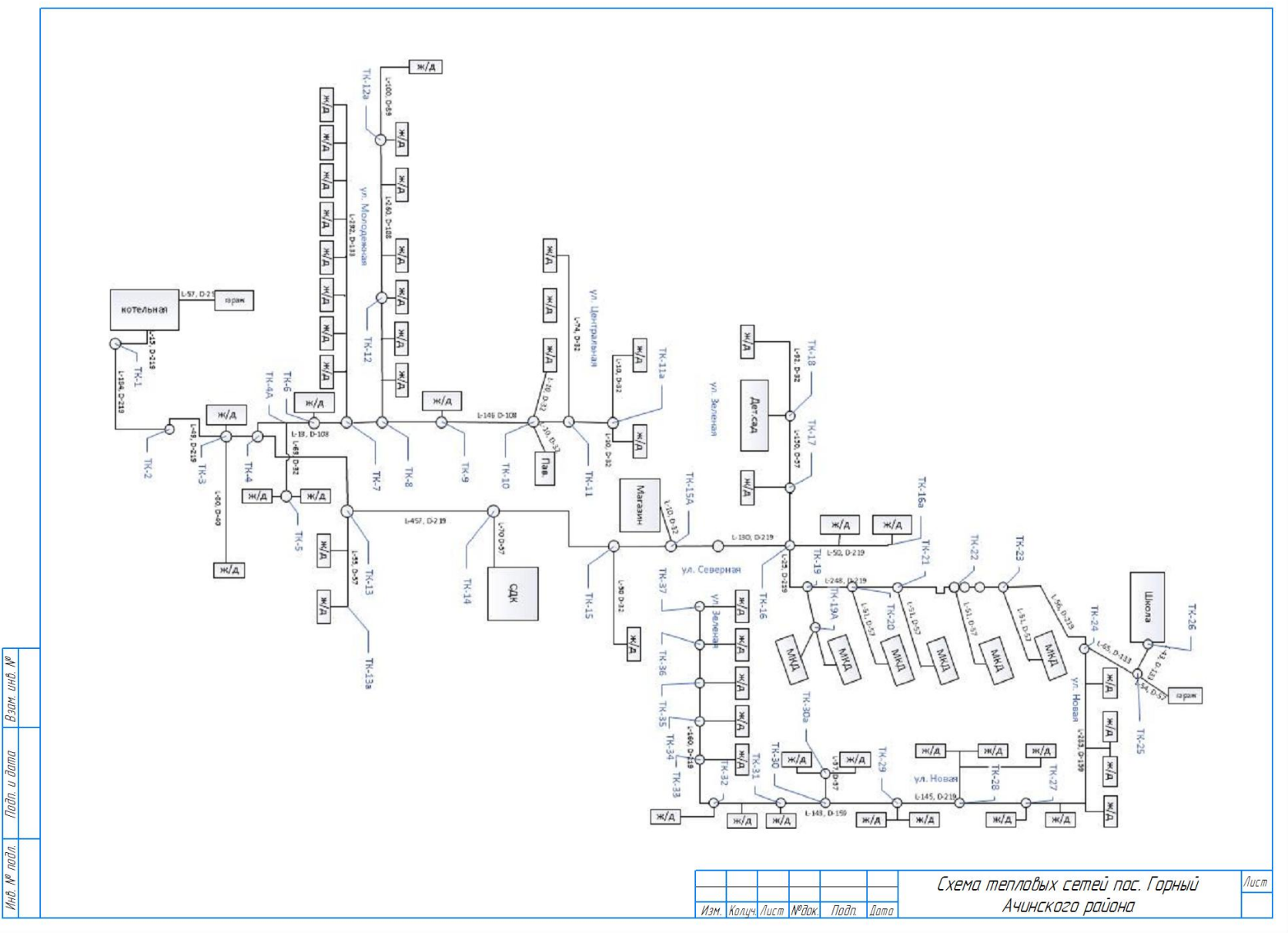
Схема тепловой сети от Котельной п. Горный – ООО «ЭнКом»
