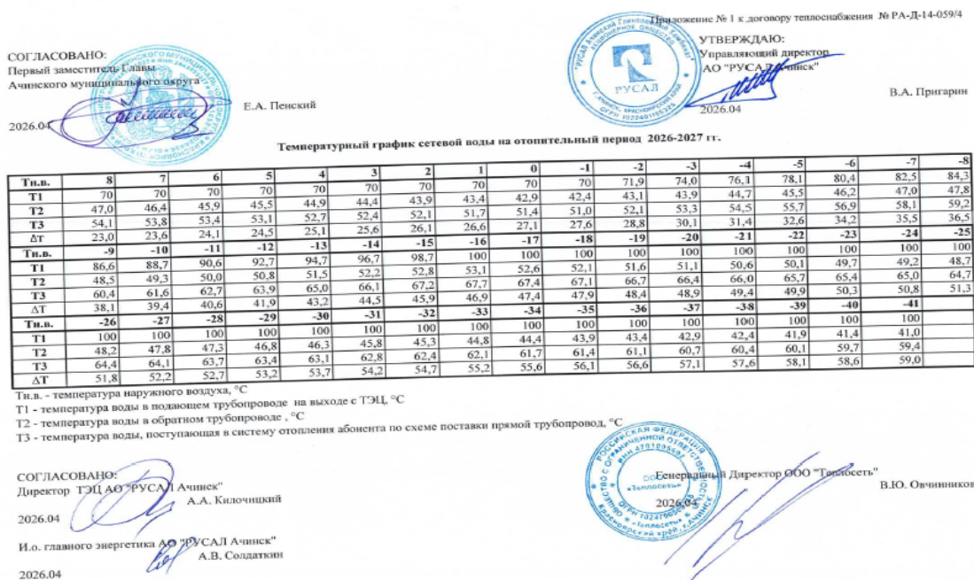
Рисунок 1.3.6.1 - График регулирования температуры сетевой воды от ТЭЦ
