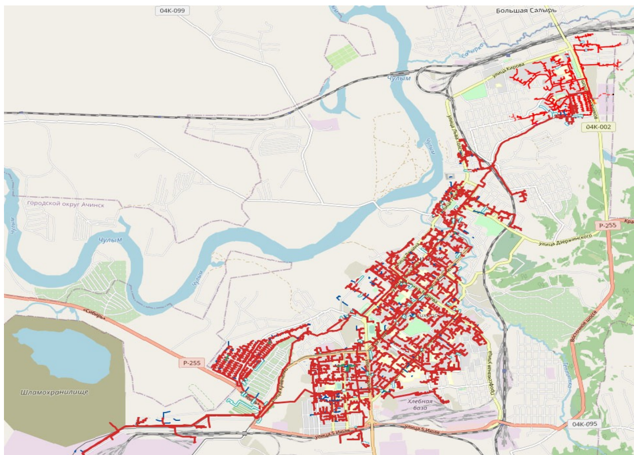
Рисунок 1.3.2.1 - Схема тепловых сетей от ТЭЦ «РУСАЛ Ачинск» и ЦТП
