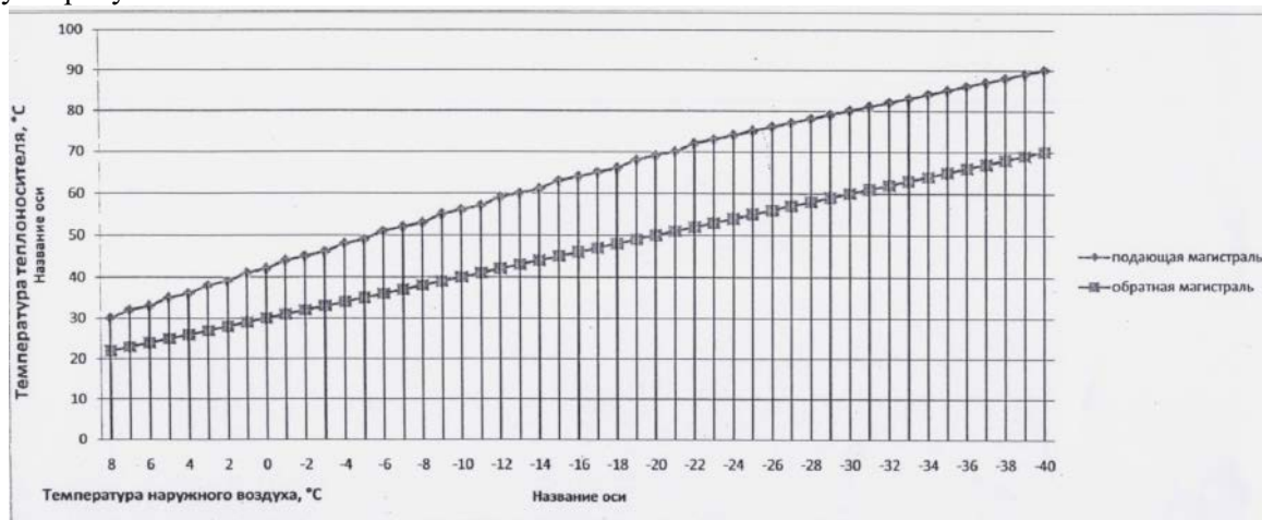
Рисунок – Температурный график для котельных ООО «ЭнКом»
