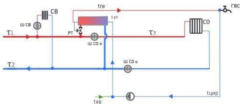
Рисунок 1.3.16.4 - Потребитель с параллельным подключением подогревателя ГВС непосредственным присоединением СО
