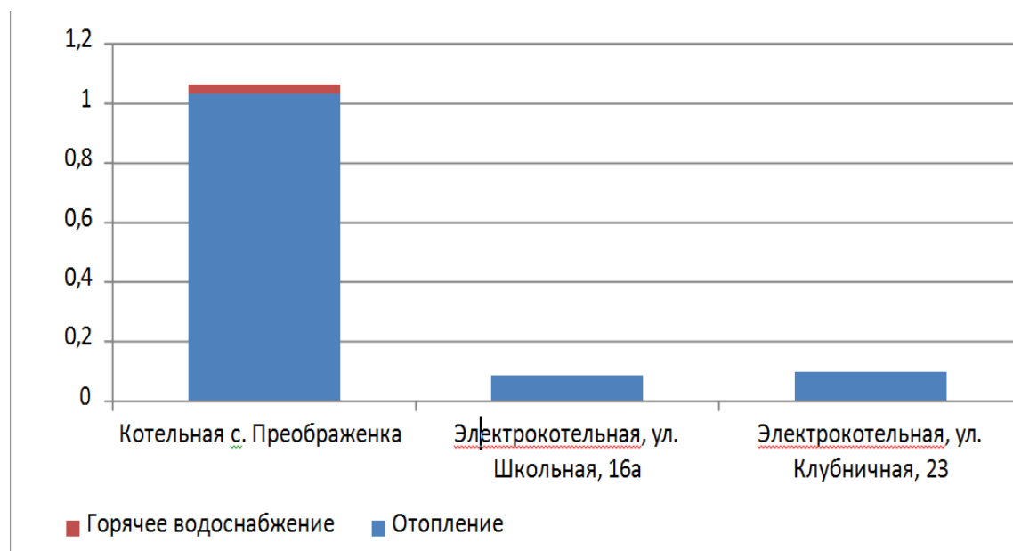
Рисунок 4. Распределение суммарных тепловых нагрузок по котельным с. Преображенка и
