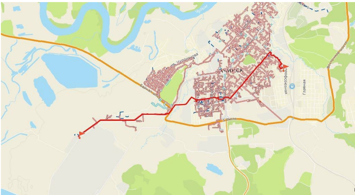
Рисунок 1.3.8.3 - Путь пьезометрического графика от ТЭЦ, 1 нитка
