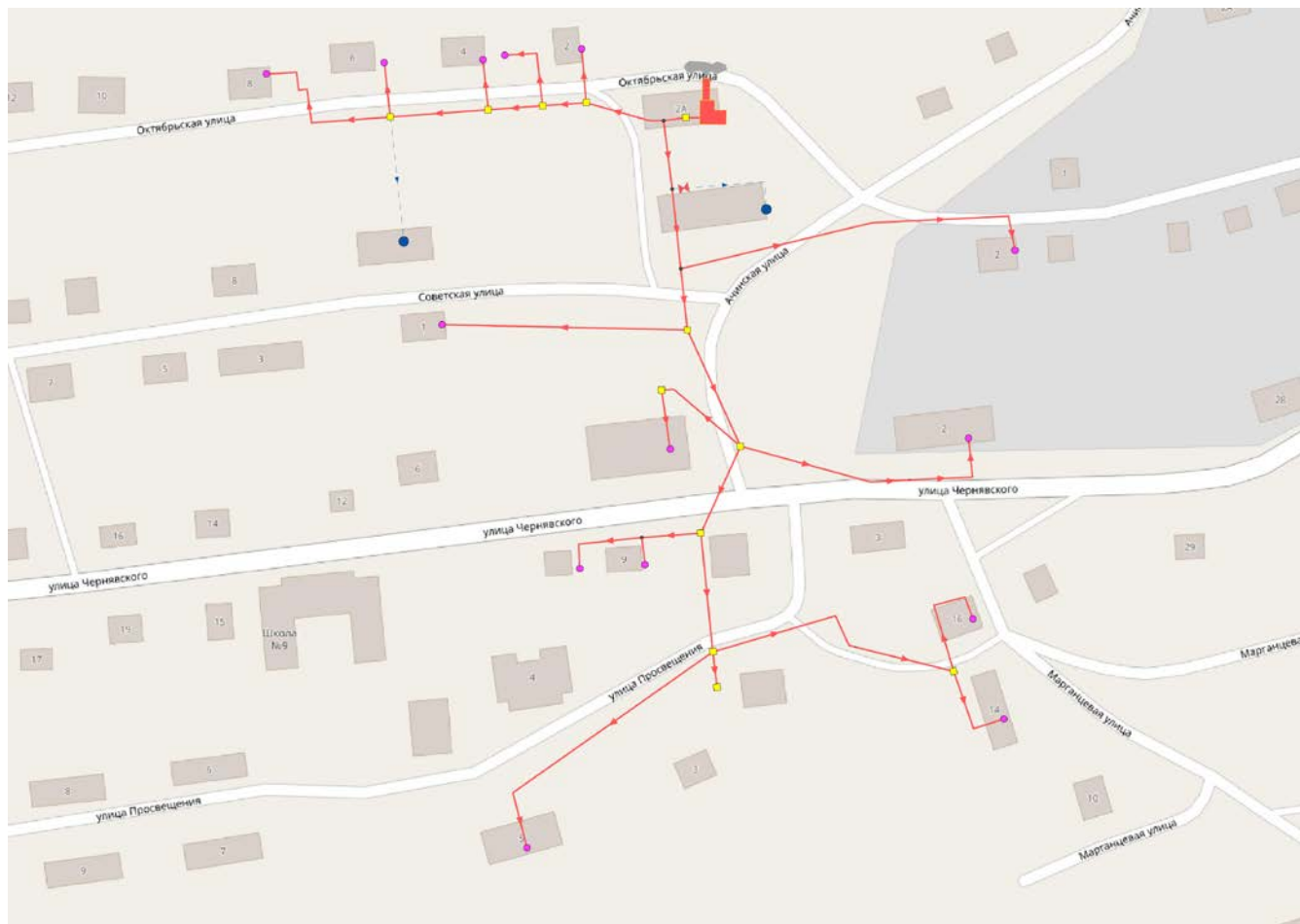
Рисунок 1.3.2.4 - Схема тепловой сети котельной № 3
