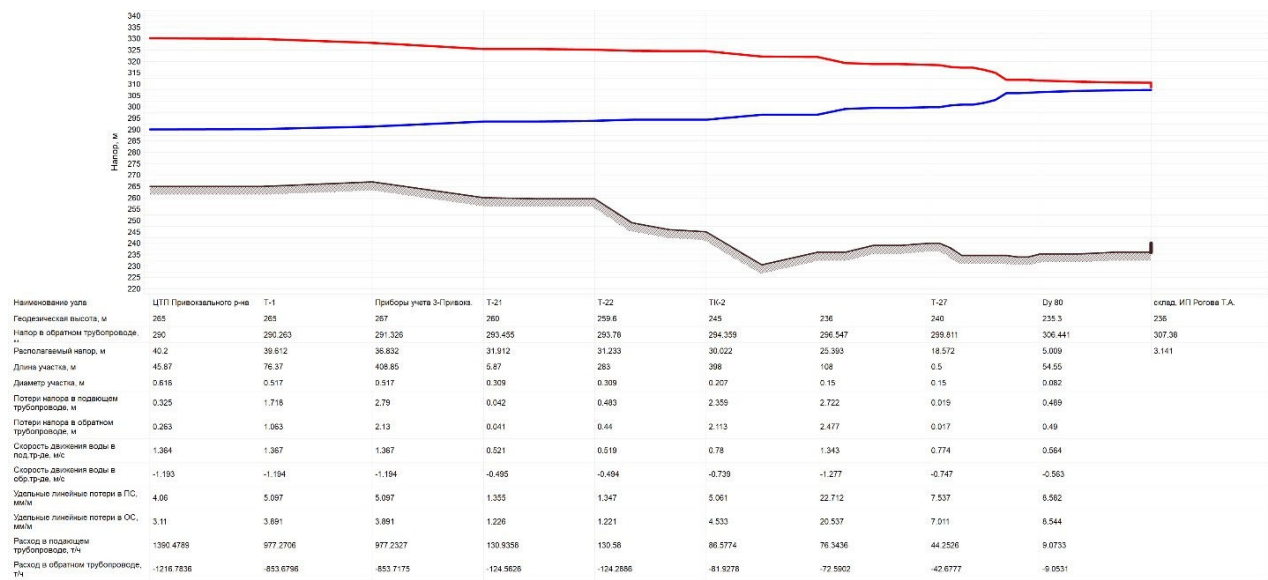
Рисунок 1.3.8.8 - Пьезометрический график от ЦТП до склада
