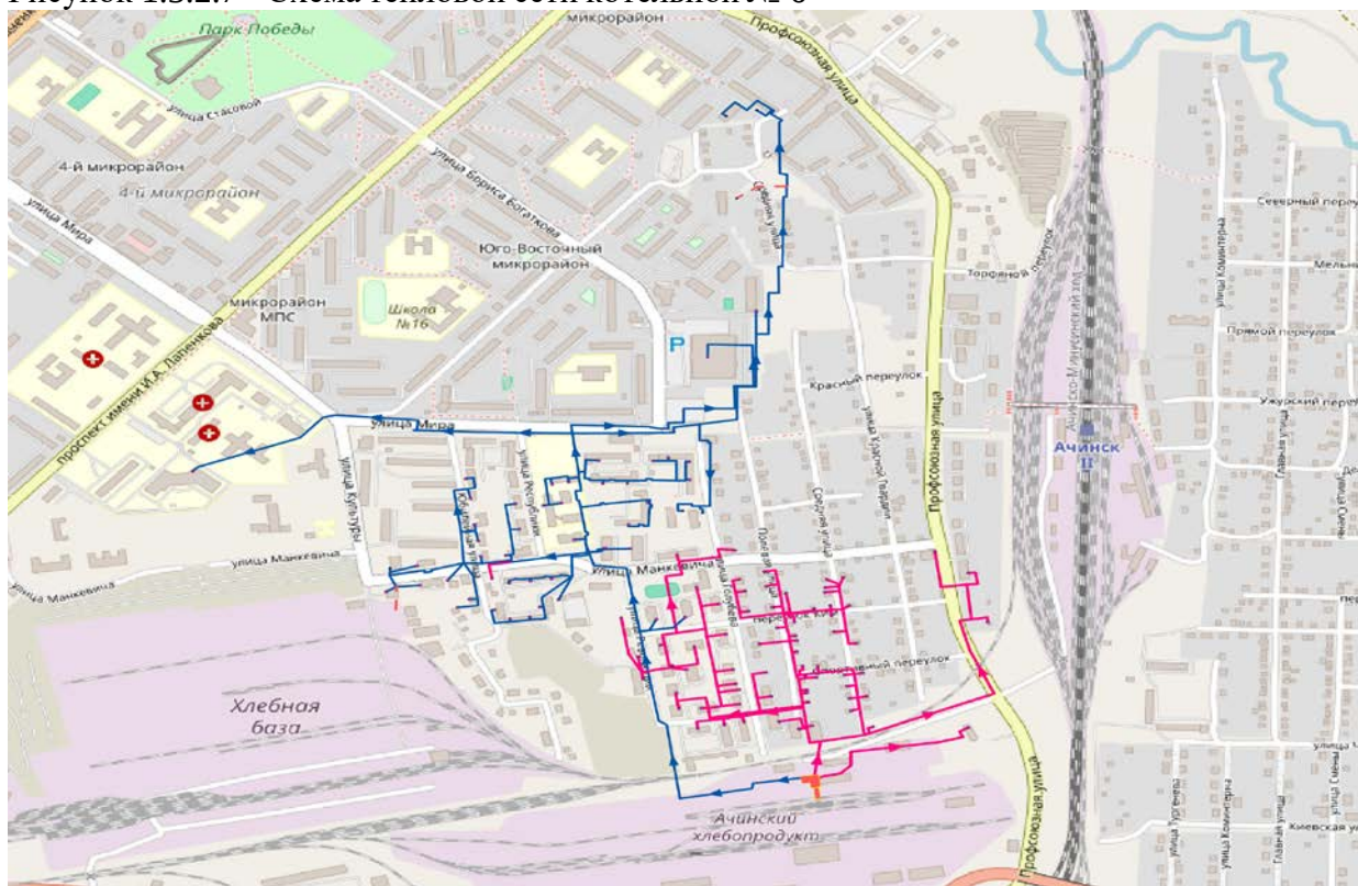
Рисунок 1.3.2.8 - Схема тепловой сети котельной ТК «Восток»
