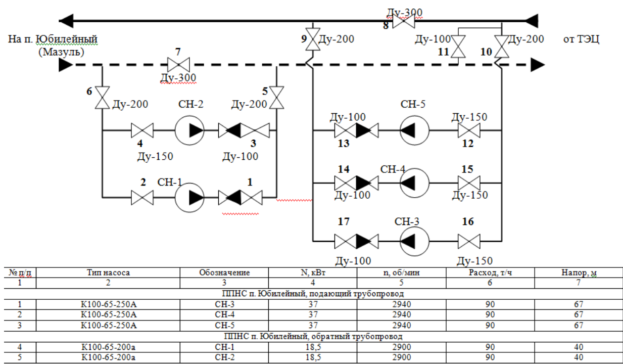
Рисунок 1.3.1.1.3- Принципиальная схема работы ПНС 2
