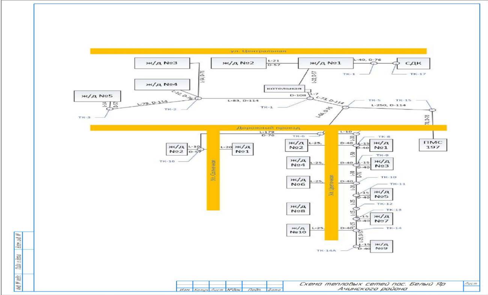
Схема тепловой сети от Котельной п. Белый Яр
