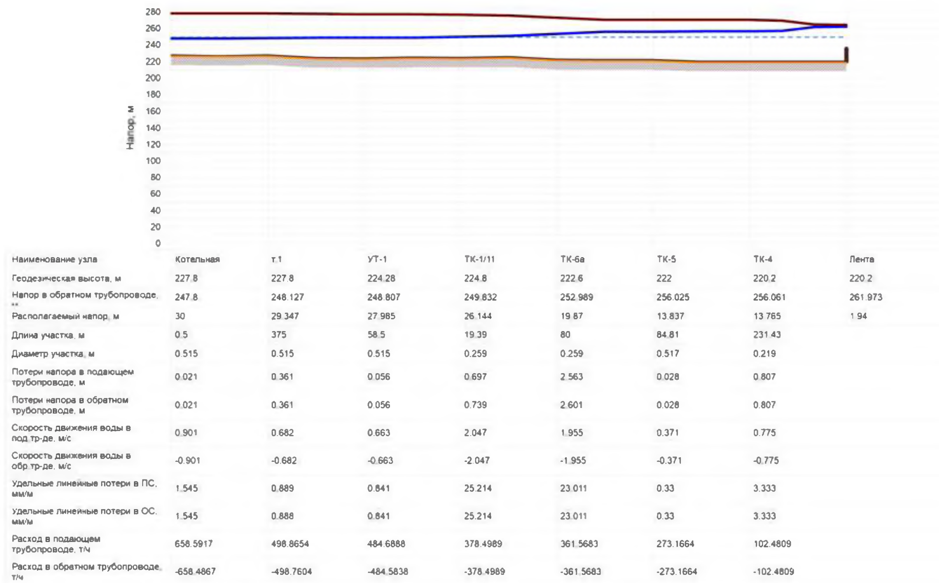
Рисунок 4.2.24. Пьезометрический график котельная ООО «ТК Восток» – супермаркет Лента
