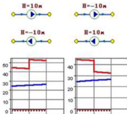
Рисунок 3.2.15. Пьезометрические графики
