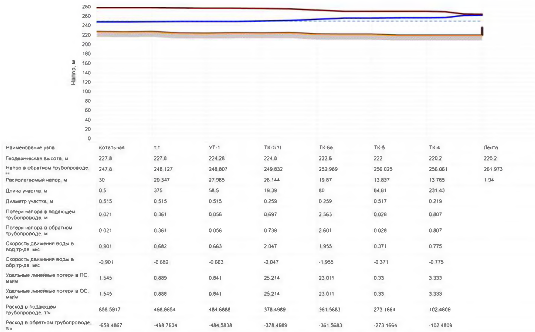
Рисунок 4.2.24. Пьезометрический график котельная ООО «ТК Восток» – супермаркет Лента
