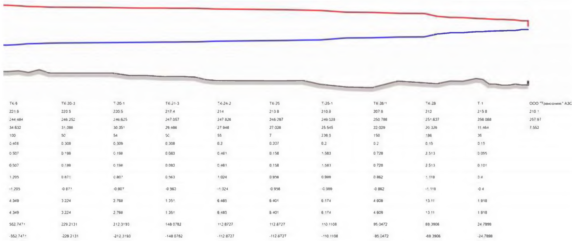
Рисунок 4.2.20. Пьезометрический график котельная №6 – АЗС
