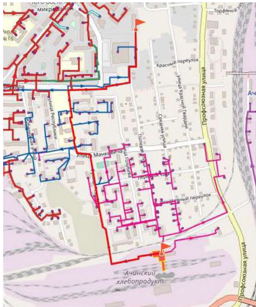
Рисунок 4.2.25. Путь построения пьезометрического графика котельная ООО «ТК Восток» – ЮВР,66
