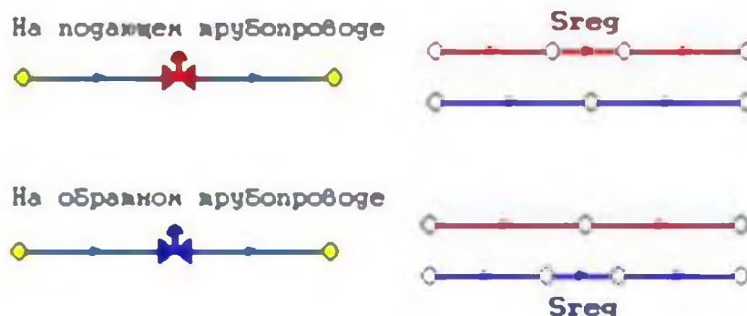
Рисунок 3.2.17. Дросселирующие устройства
