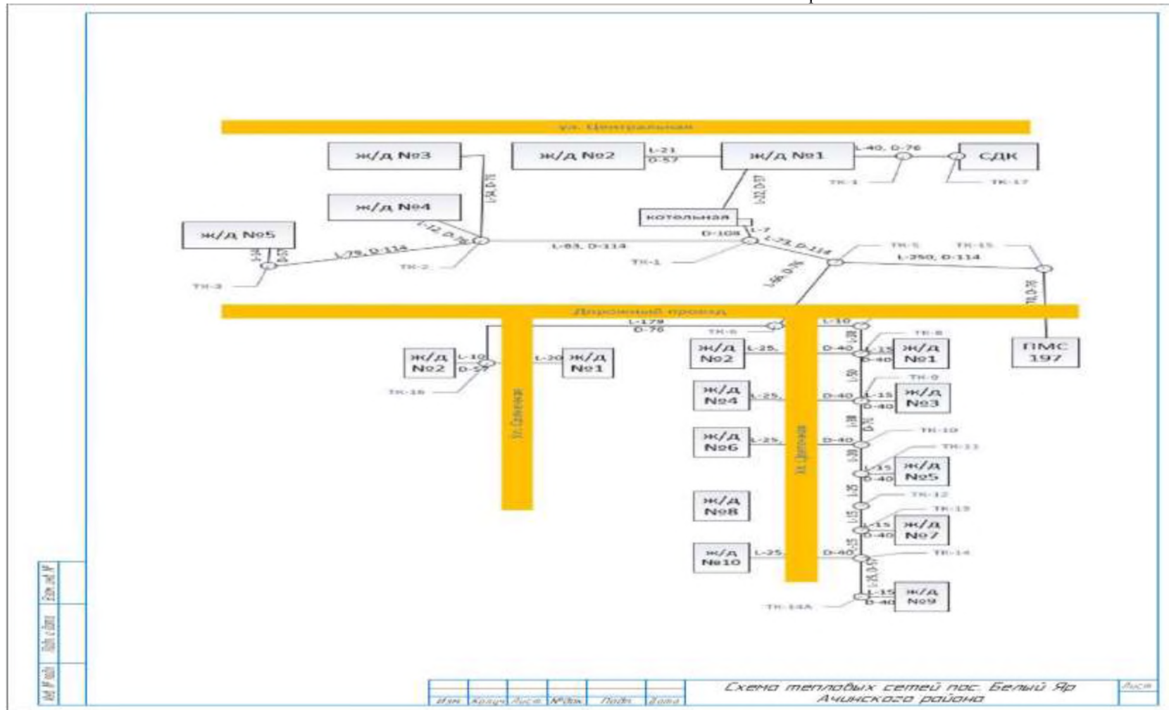
Схема тепловой сети от Котельной с. Белый Яр
