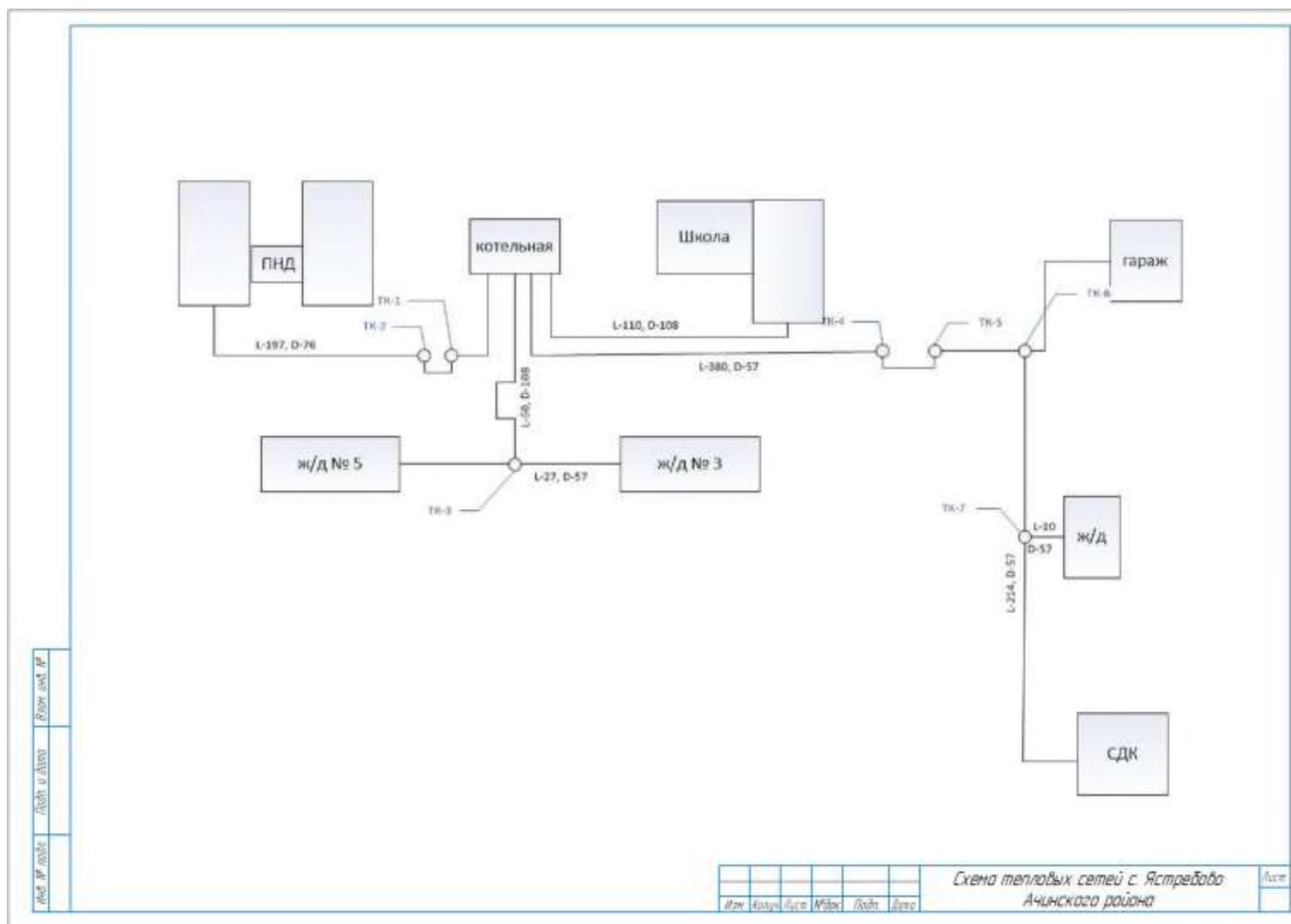
Схема тепловой сети от Котельной с. Ястребово
