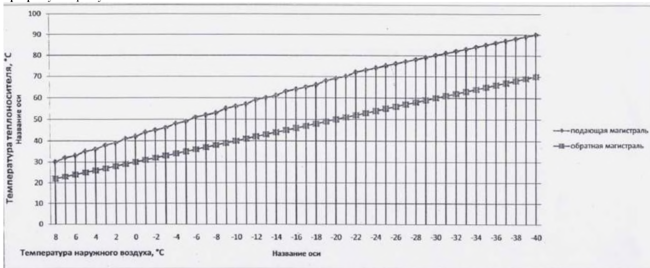
Рисунок – Температурный график для котельных ООО «ЭнКом»
