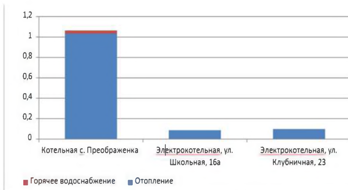
Рисунок 4. Распределение суммарных тепловых нагрузок по котельным с. Преображенка и с. Большая Салырь
