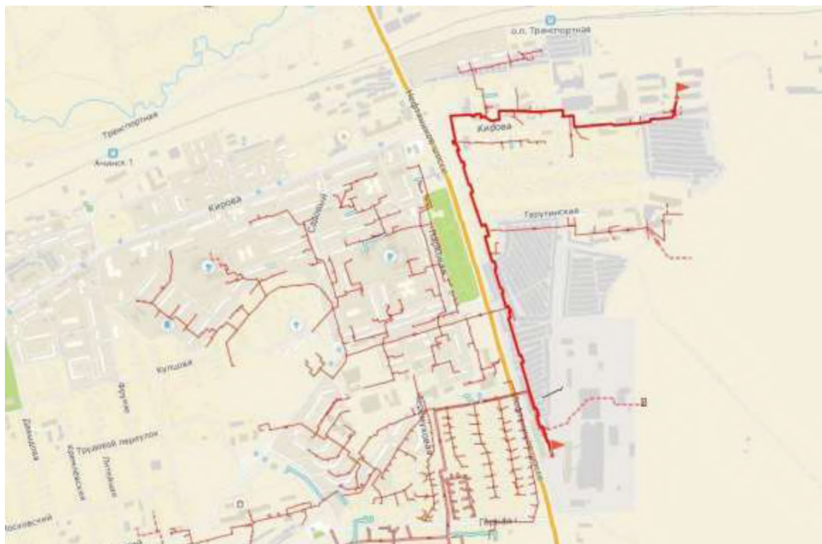
Рисунок 1.3.8.7 - Путь пьезометрического графика от ЦТП до склада
