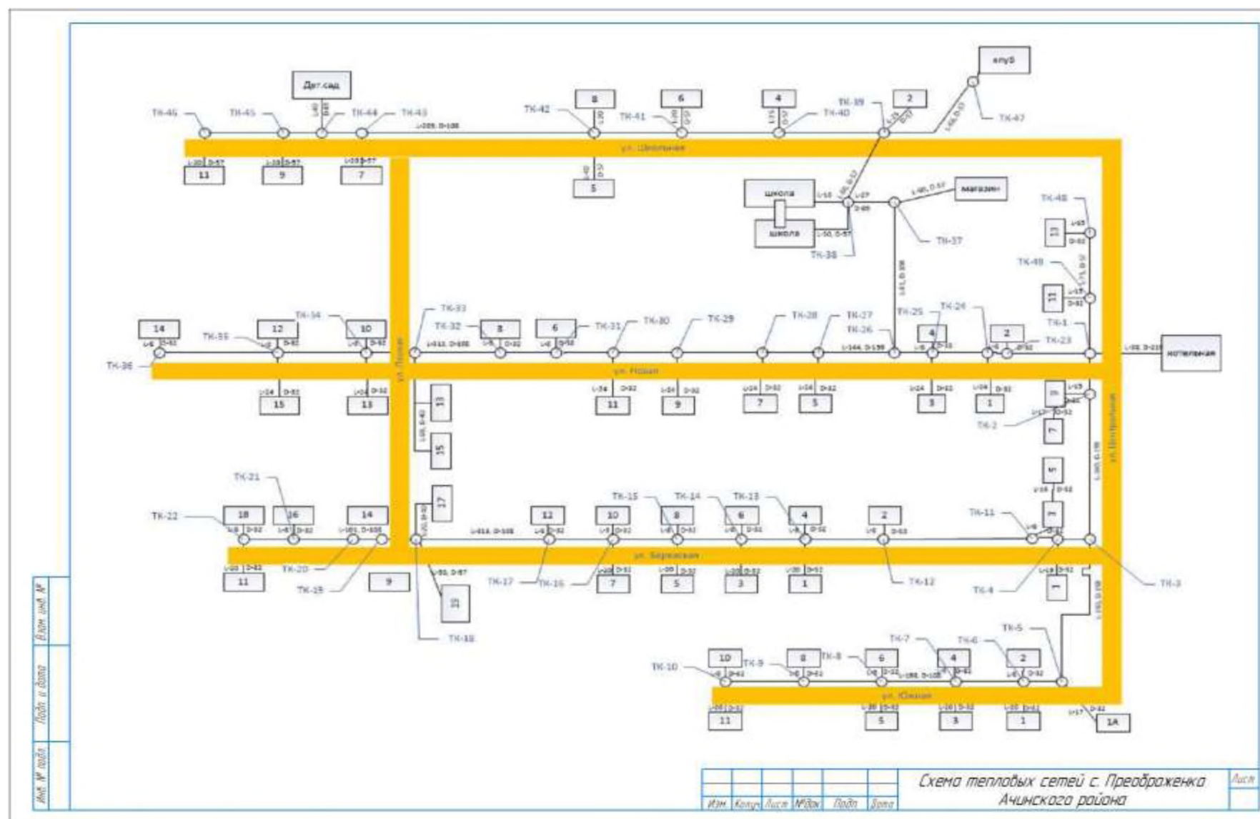
Схема тепловой сети от Котельной с. Преображенка
