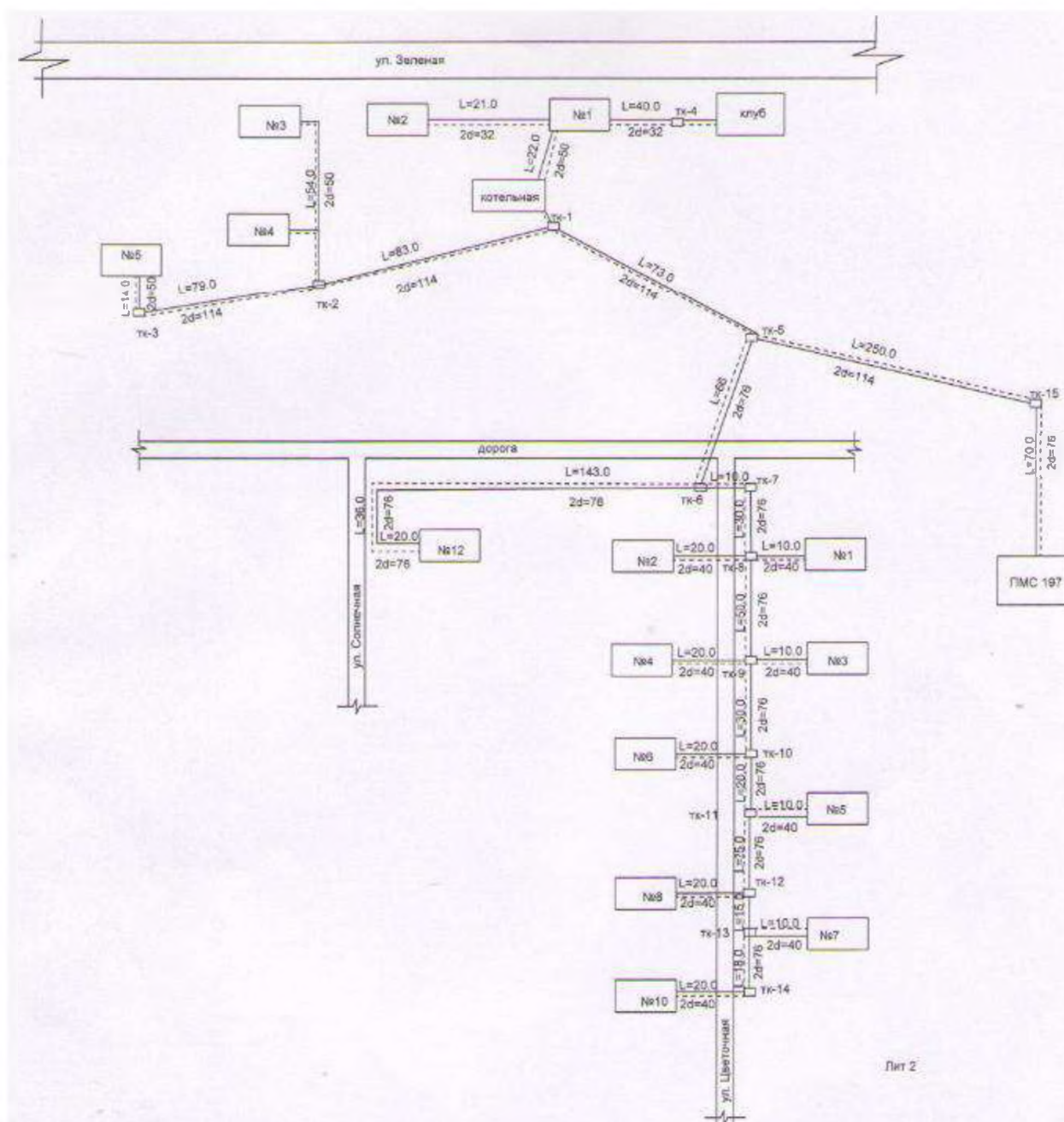
Рисунок - Зона действия котельной, ул. ПМС, 1а
