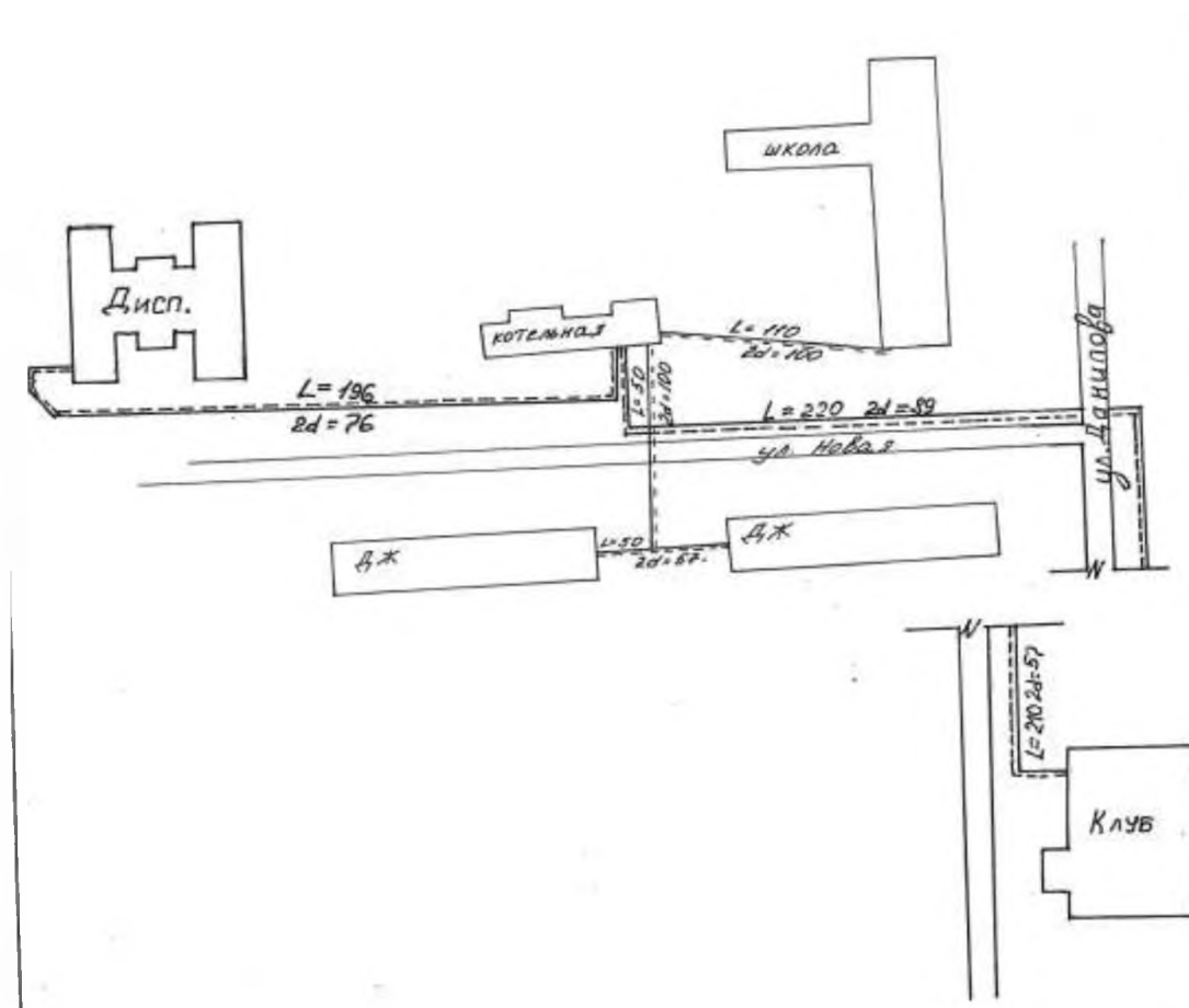
Рис унок 1.3.26.2.1 - Схема тепловой сети.
