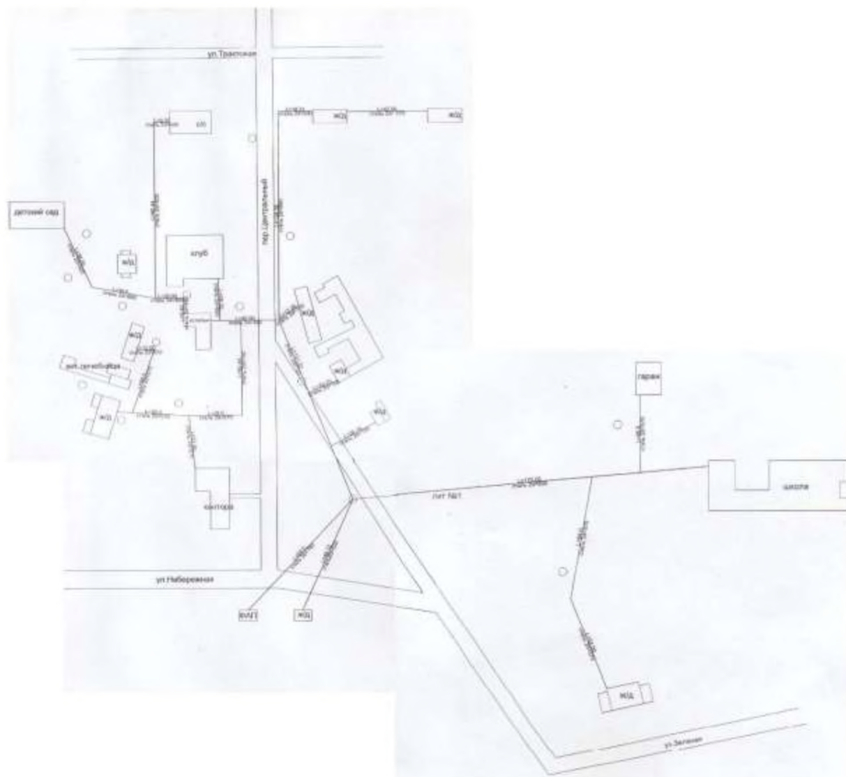
Рисунок - Зона действия котельной, пер. Центральный, 4а
