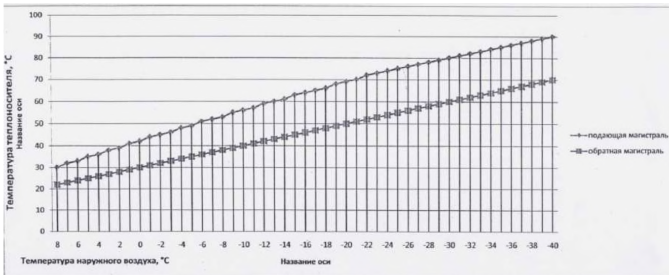
Рисунок 1.3.20.6.1 – Температурный график для котельных ООО «ЭНКОМ»
