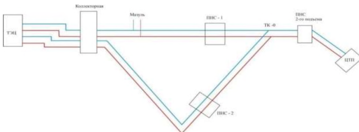
Рисунок 1.3.1.1.- Принципиальная схема магистральных тепловых сетей от Ачинской ТЭЦ.
