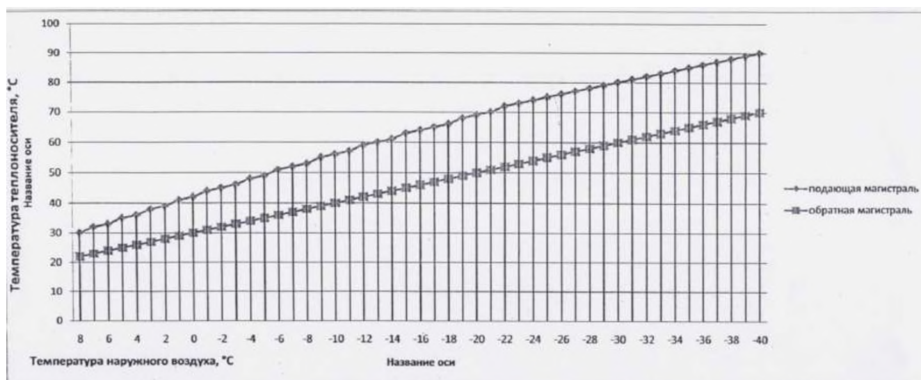
Рисунок 1.3.26.6.1 – Температурный график для котельных ООО «ЭнКом»
