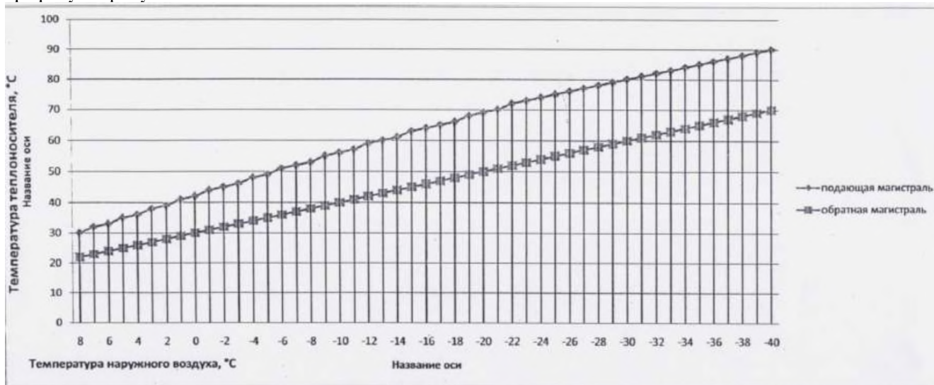
Рисунок 1.3.24.6.1 – Температурный график для котельных ООО «ЭнКом»
