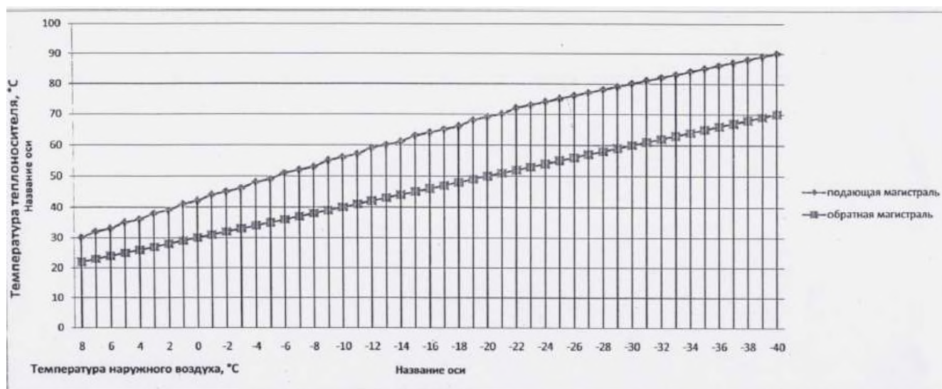
Рисунок 1.3.21.6.1 – Температурный график для котельных ООО «ЭнКом»
