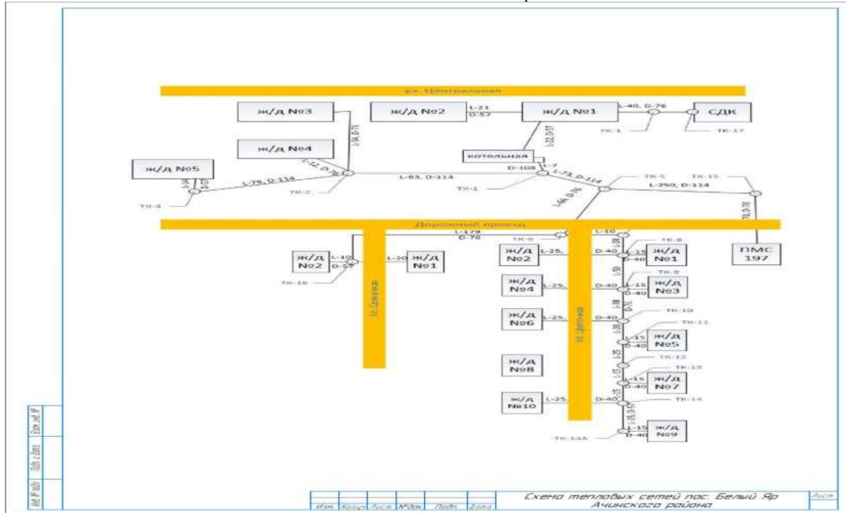
Схема тепловой сети от Котельной с. Белый Яр – ООО «ЭнКом»
