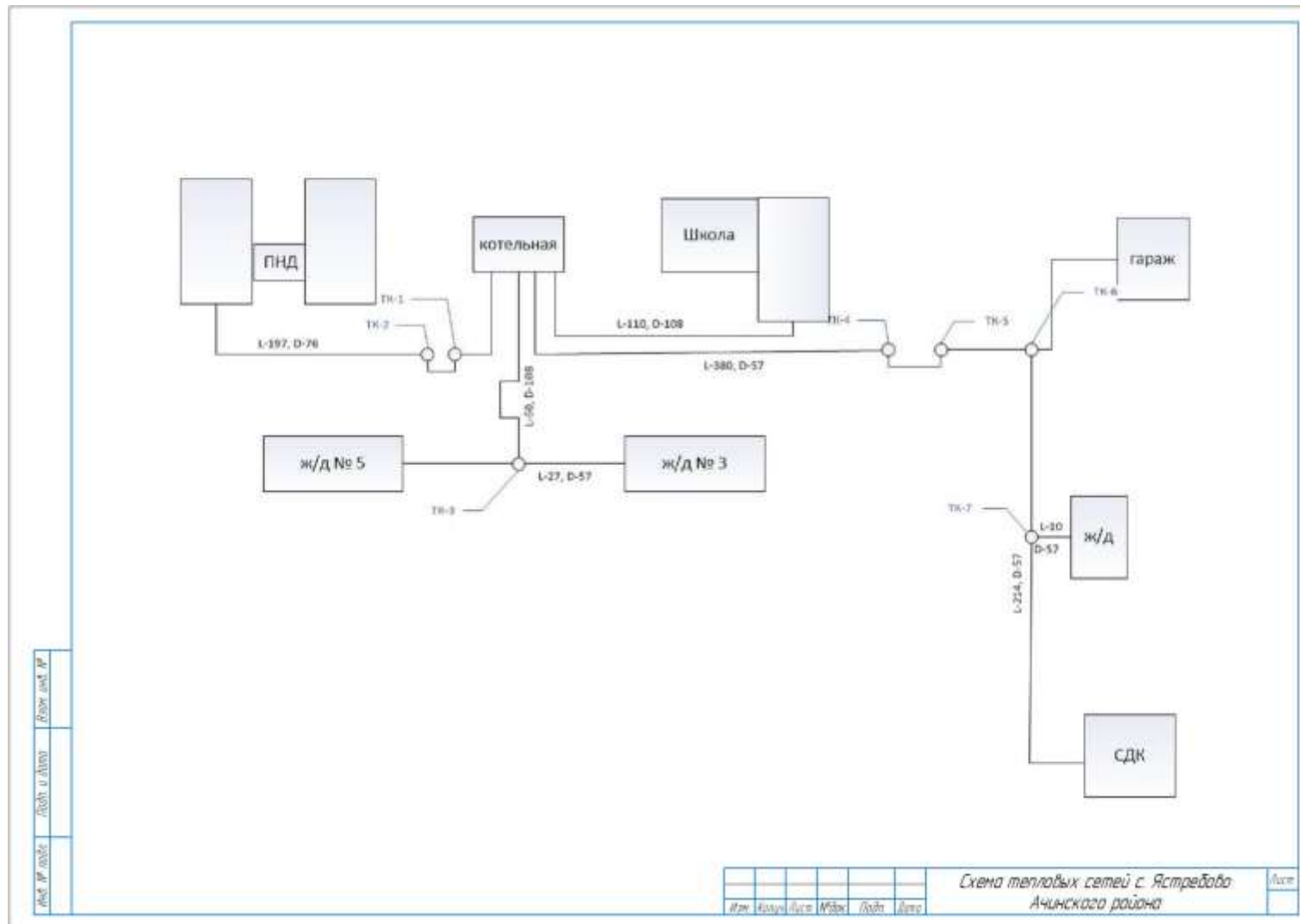
Схема тепловой сети от Котельной с. Ястребово – ООО «ЭнКом»
