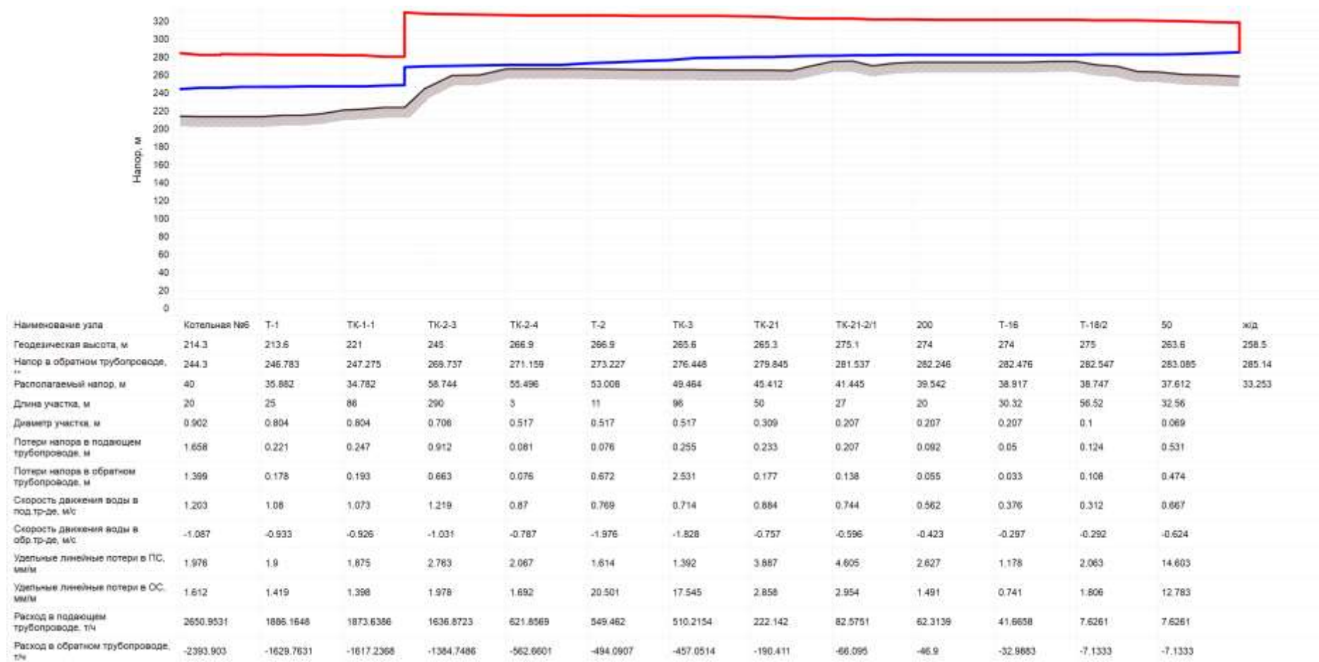
Рисунок 4.2.22. Пьезометрический график котельная № 6 – жилой дом в Привокзальном районе
