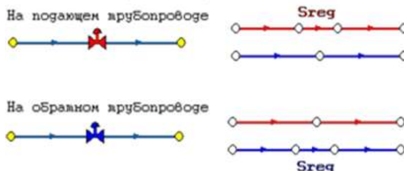
Рисунок 3.2.17. Дросселирующие устройства
