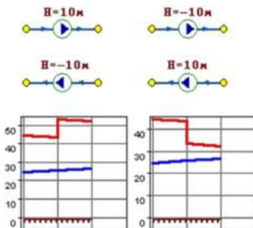
Рисунок 3.2.15. Пьезометрические графики
