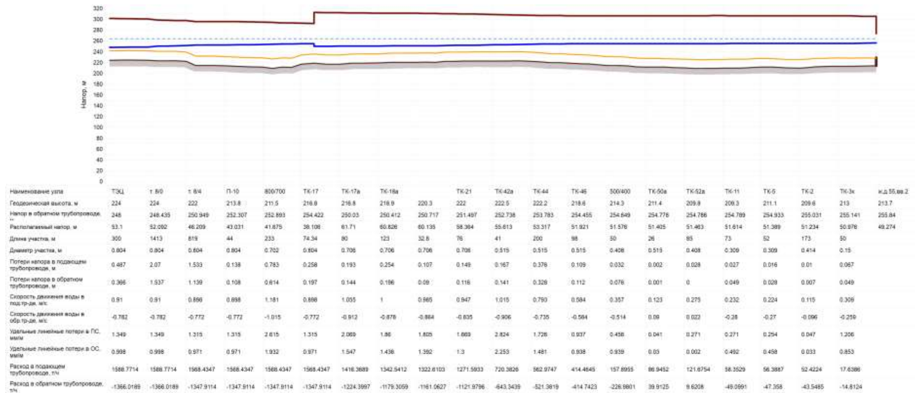
Рисунок 4.2.10. Пьезометрический график ТЭЦ АО «РУСАЛ Ачинск» 1-ая нитка
