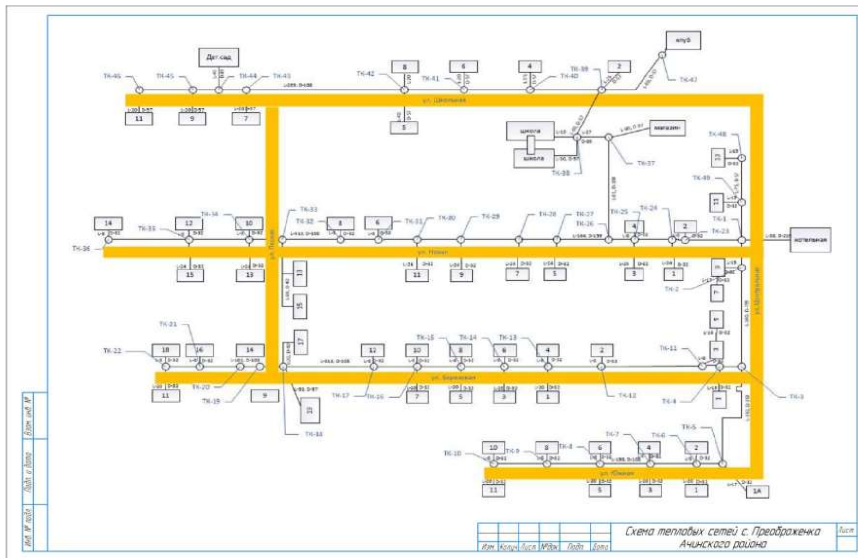
Схема тепловой сети от Котельной с. Преображенка – ООО «ЭнКом»
