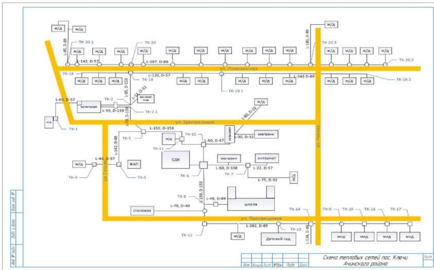
Схема тепловой сети от Котельной п. Ключи – ООО «ЭнКом»
