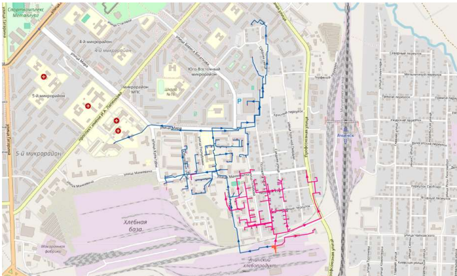
Рисунок 4.2.5. Перспективная схема сетей котельной ООО «ТК Восток»
