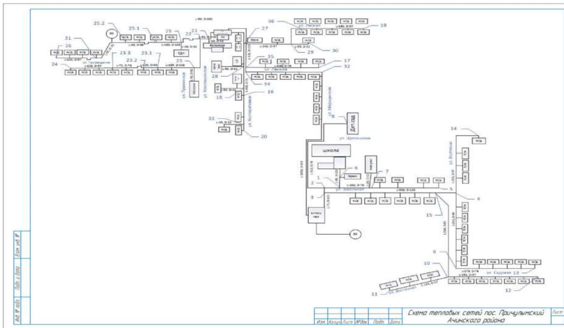
Схема тепловой сети от Котельной п. Причулымский- ООО «ЭнКом»
