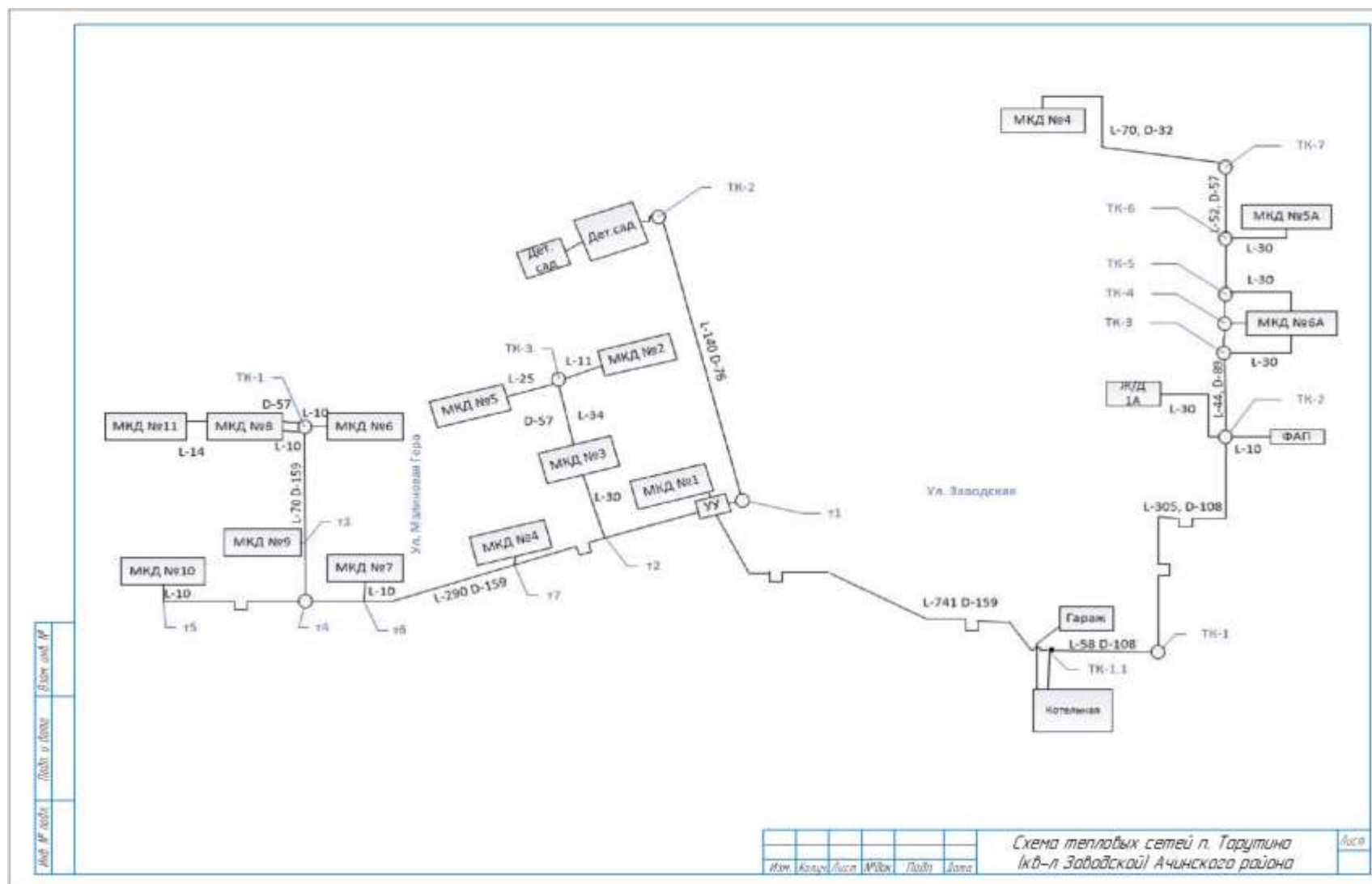
Схема тепловой сети от Котельной п. Тарутино - ООО «ЭнКом»
